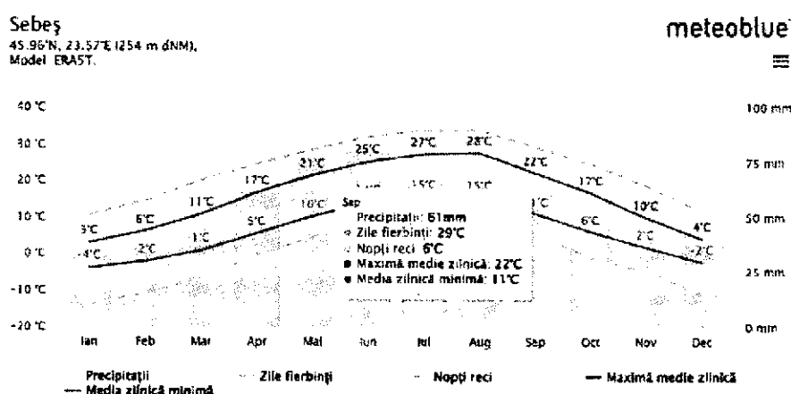
Temperatura și precipitațiile medii
