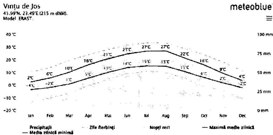
Fig.4 Temperatura și precipitații medii Vințu de Jos 9
