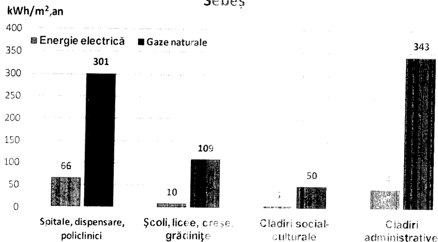
Distribuția consumului specific de energie pe principalele tipuri de clădiri municipale în 2016 în Mun. Sebeș
