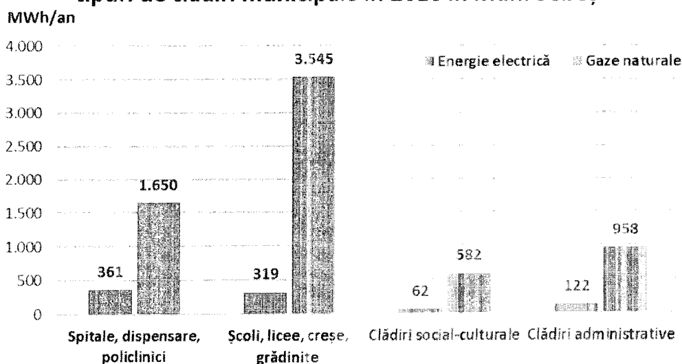
Distribuția consumului de energie pe principalele tipuri de clădiri municipale în 2016 în Mun. Sebeș
